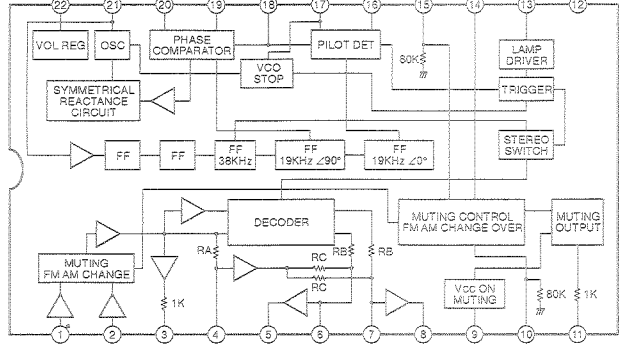
MPX
