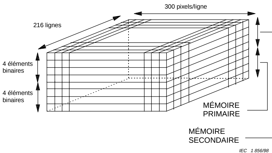
Figure F.1b – Un plan de mémoire à 256 couleurs
