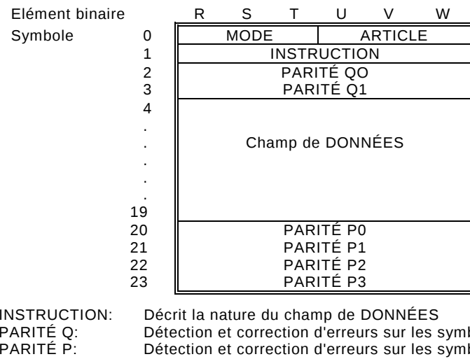
Figure 20 – Organisation générale d'un ENSEMBLE
