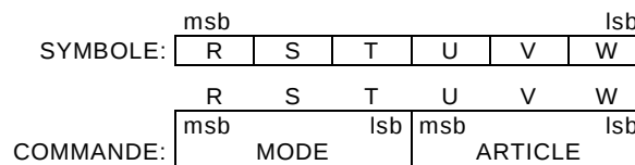
Figure 19 – Format de base pour les voies R à W de signalisation
