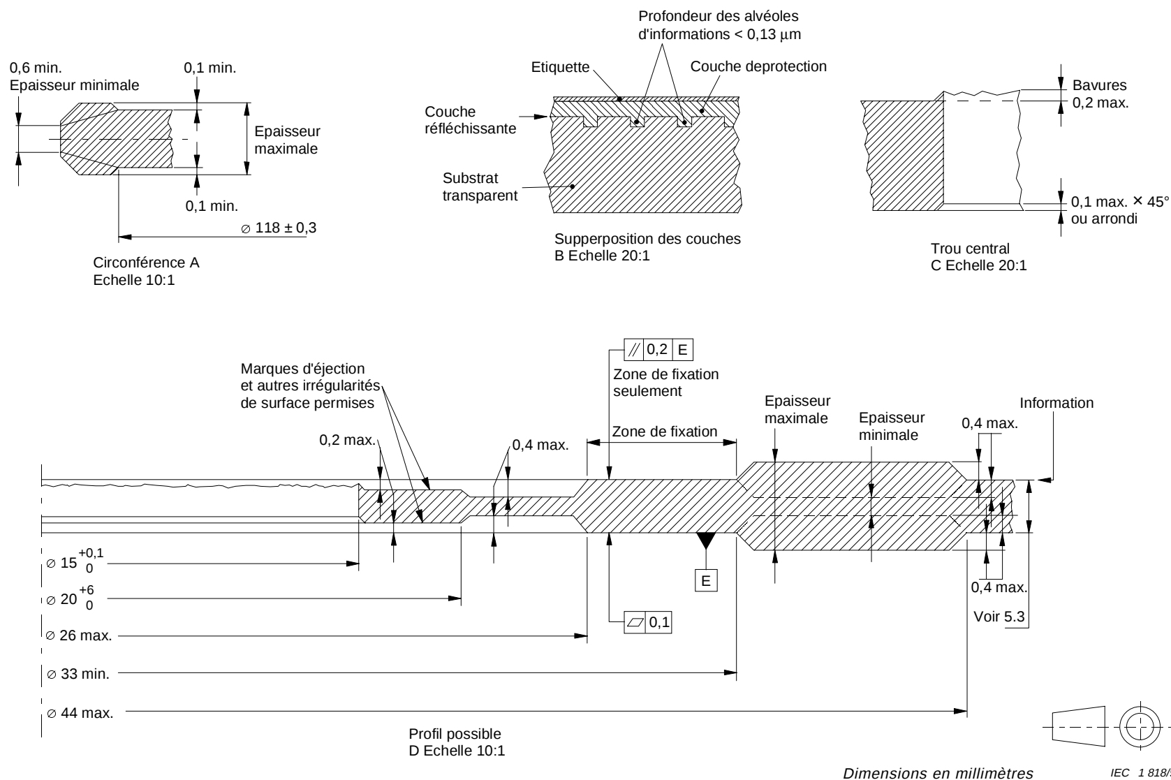
Figure 2b – Dimensions du disque
