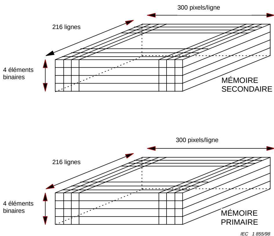
Figure F.1a – Deux plans de mémoire à 16 couleurs
