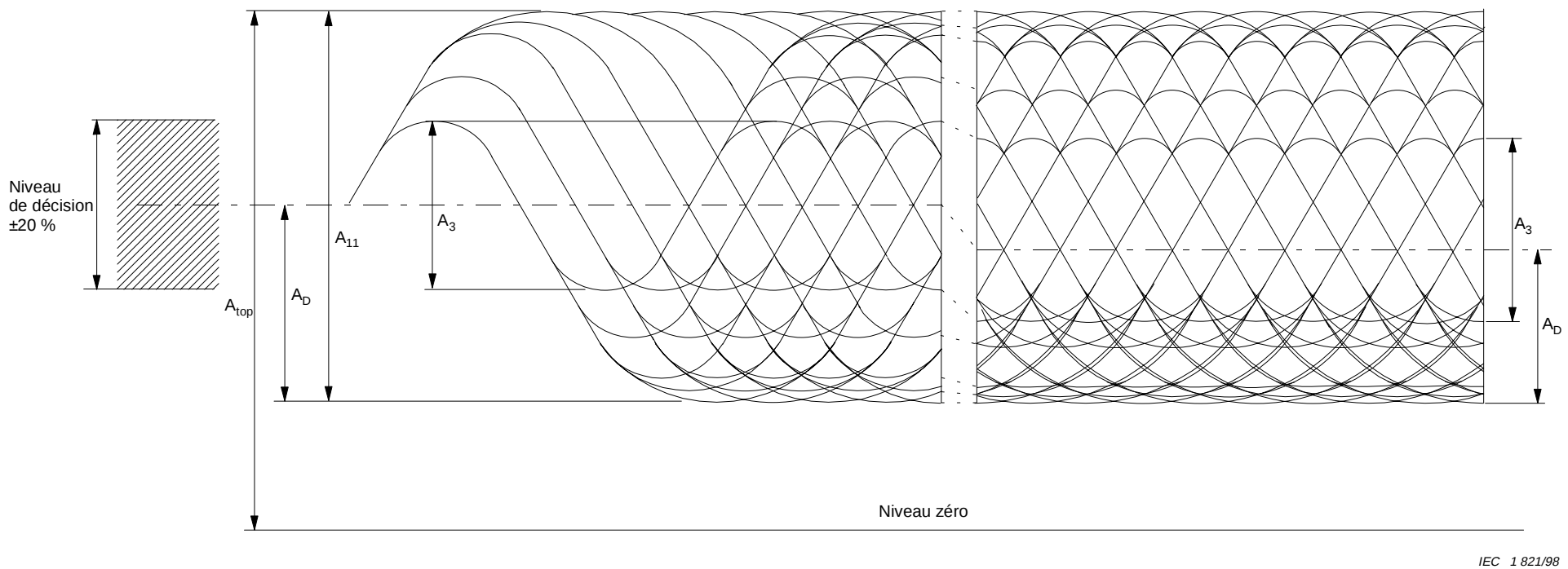
Figure 3 – Signal haute fréquence
