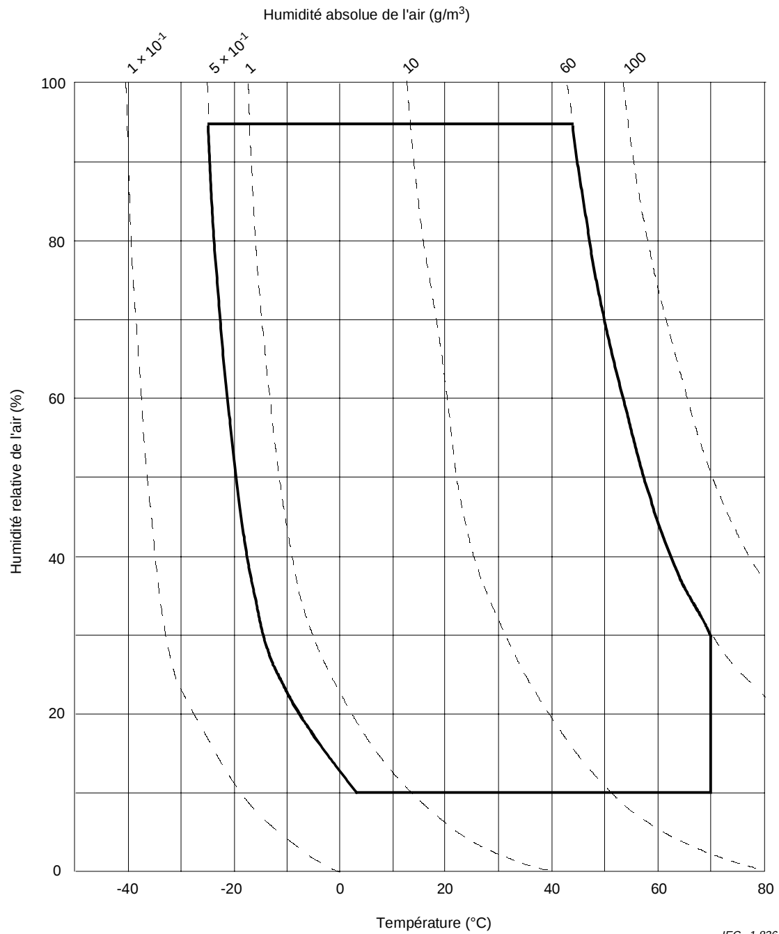
Figure 17 – Conditions de fonctionnement du disque
